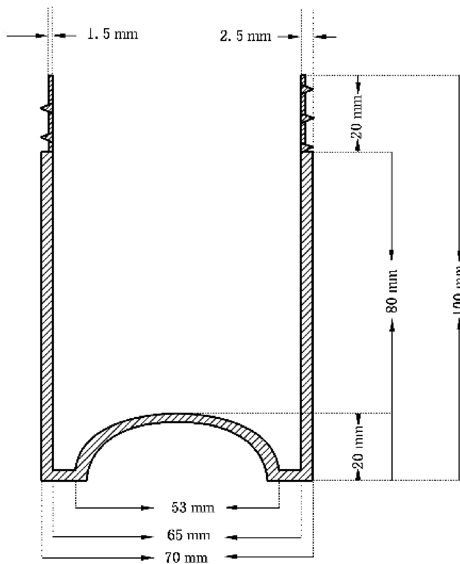
a) 诱蚊诱卵器平面尺寸
