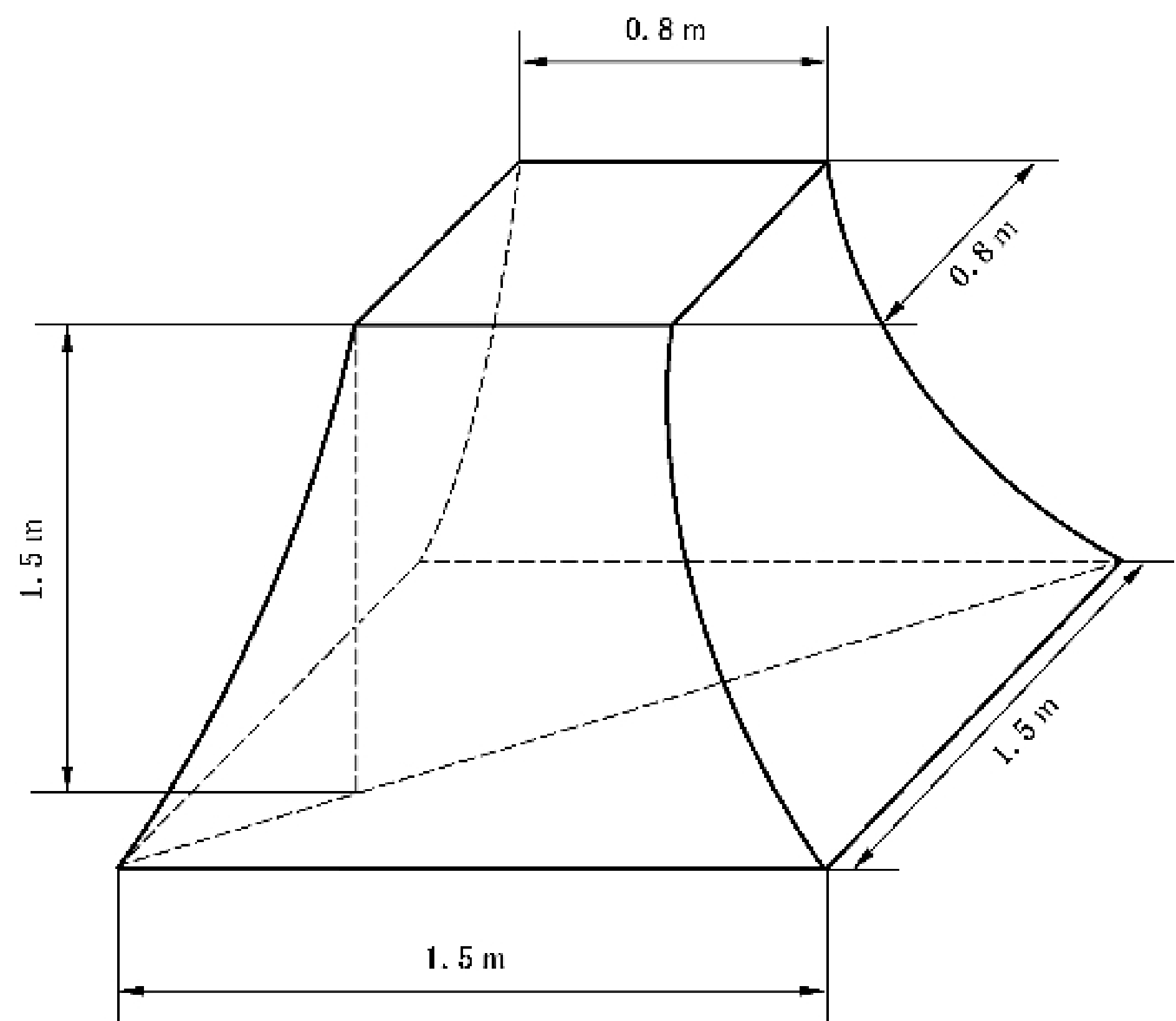
图 B.3 诱蚊帐示意图
